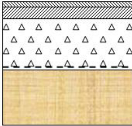
Конструкция д.о. подъездной дороги
