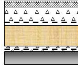
Конструкция д.о. контейнерной площадки
